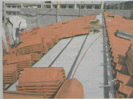
瓦屋根の施工例。黒い桧木の上に瓦を固定していく。屋根と瓦のすき間が空気層になる
